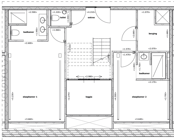
Plattegrond verdieping 03 1:50
