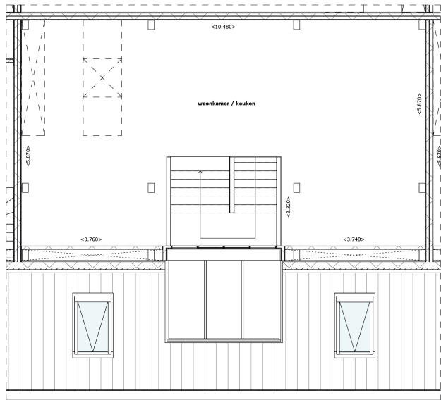
Plattegrond verdieping 04 1:50
